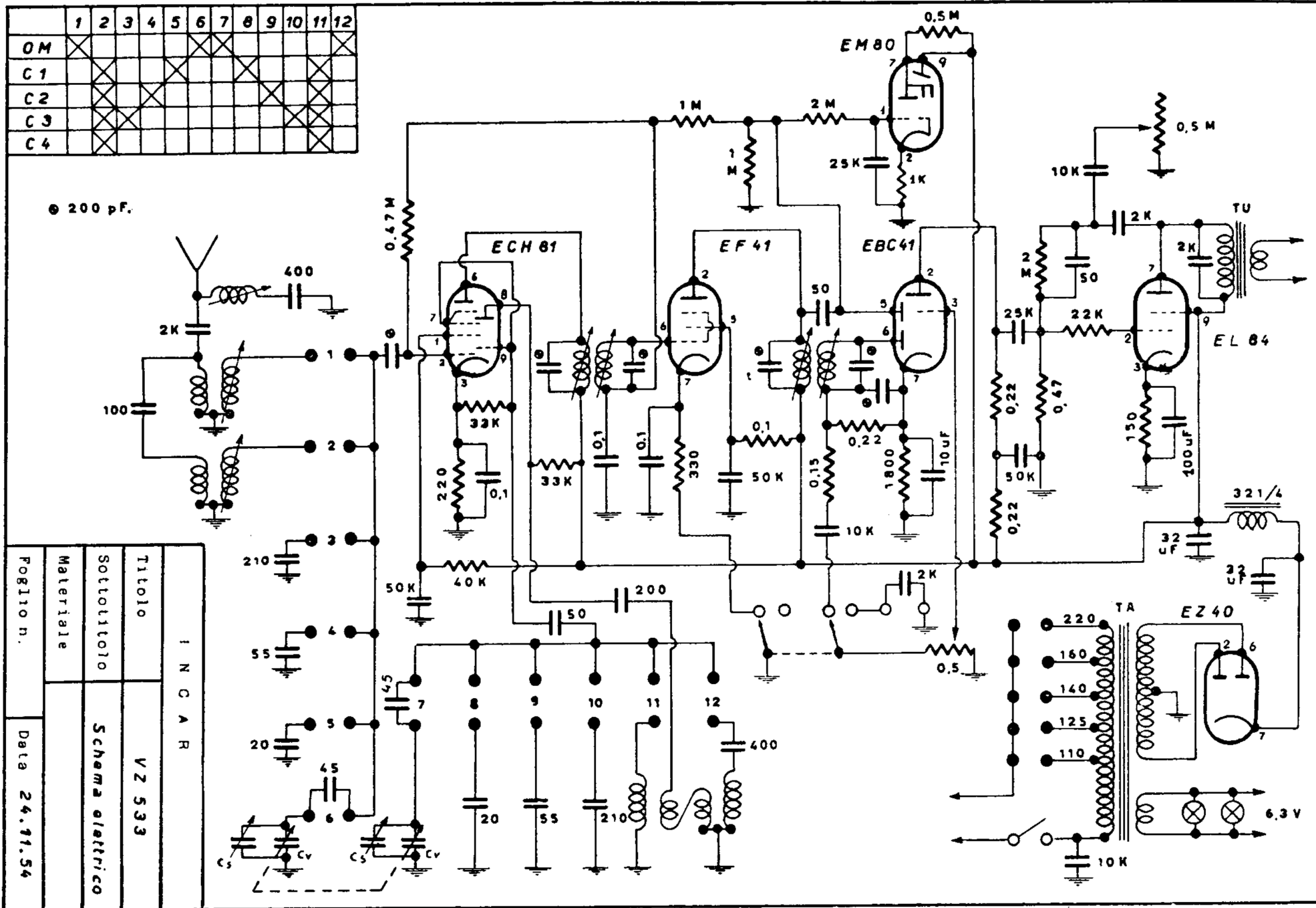
INCAR - Mod. VZ 533. Ricevitore a onde medie con quattro bande allargate in onde corte. Potenza d'uscita 3 watt. Consumo 50 watt.
